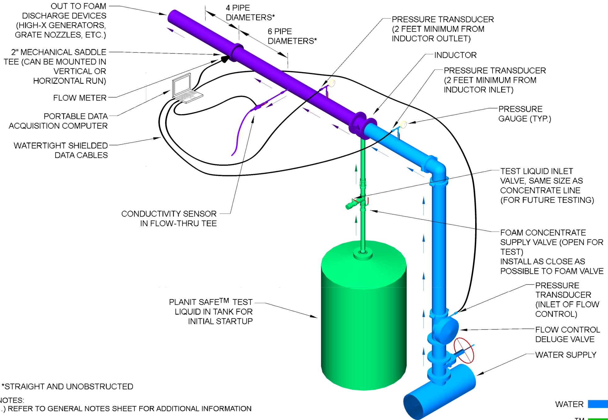
Drawing - VFTDW215 2019-04-01
