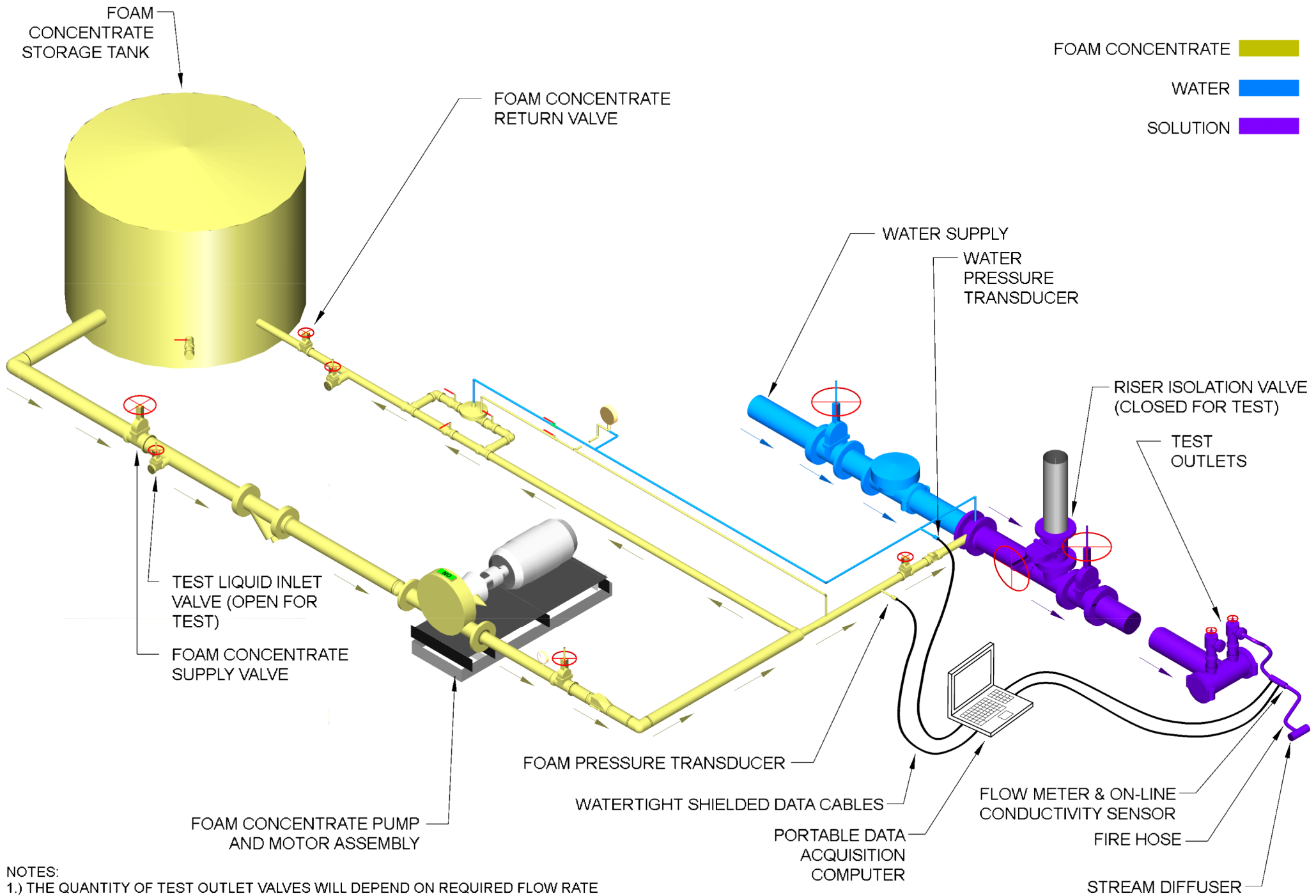
Drawing - VFTDW101 REV. A 2018-12-14
